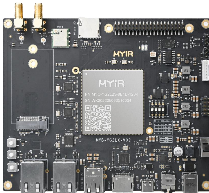
图 1-1 MYD-YG2LX 开发板
