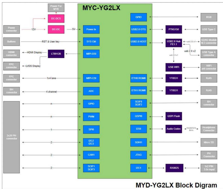
图 4-3 MYD-YG2LX 开发板系统框架图
