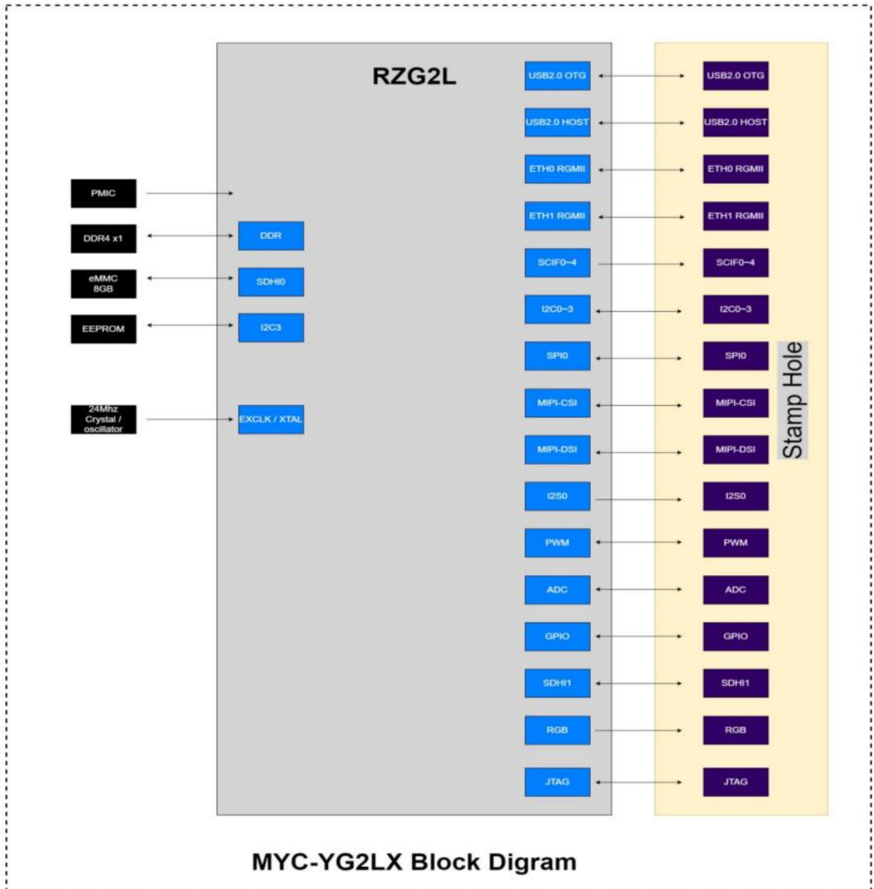
图 3-3 MYC-YG2LX 核心板系统框图
