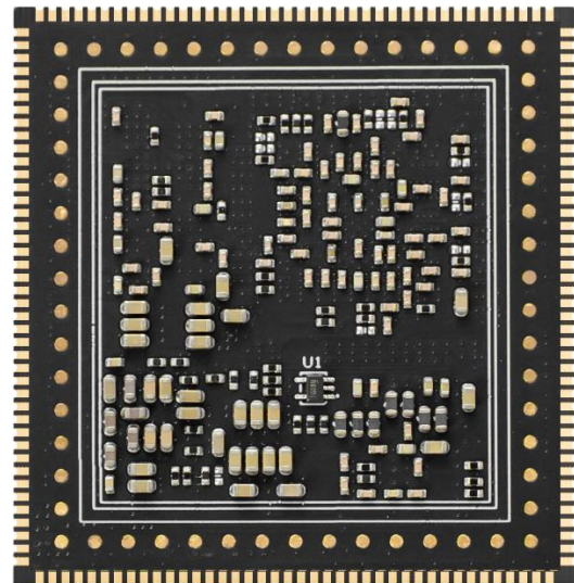
图 3-2 核心板 MYC-YG2LX 背面图
