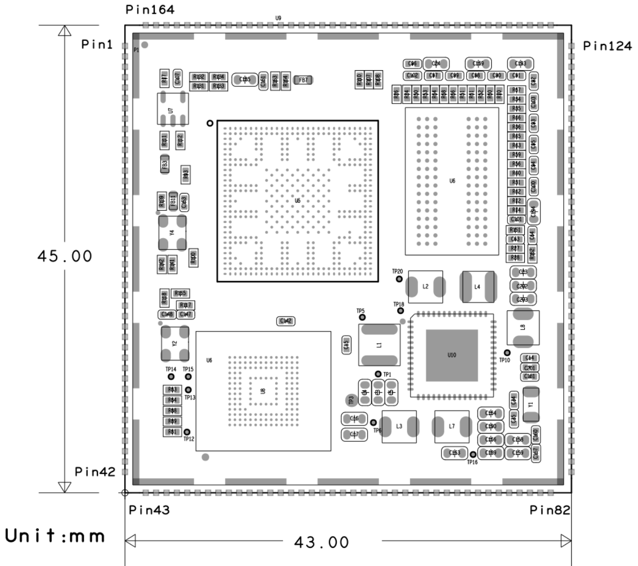
图 3-4 MYC-YG2LX 核心板机械结构图 (单位: mm)
