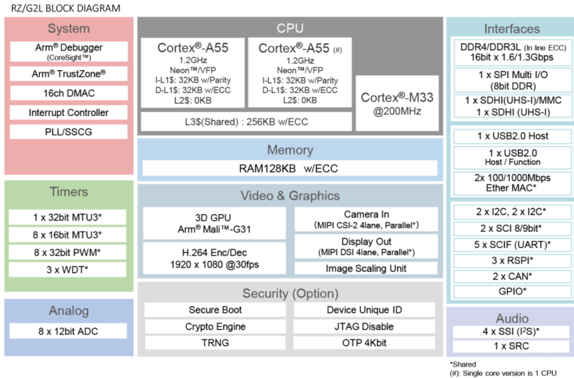
图 2-1 RZ/G2L 处理器框图
