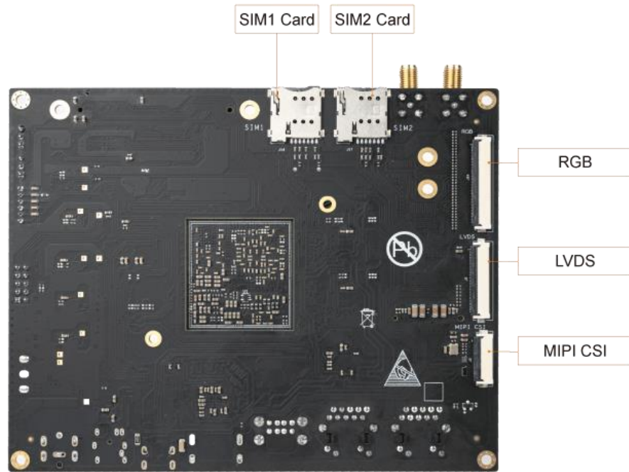
图 4-2 MYD-YG2LX 开发板接口背面图
