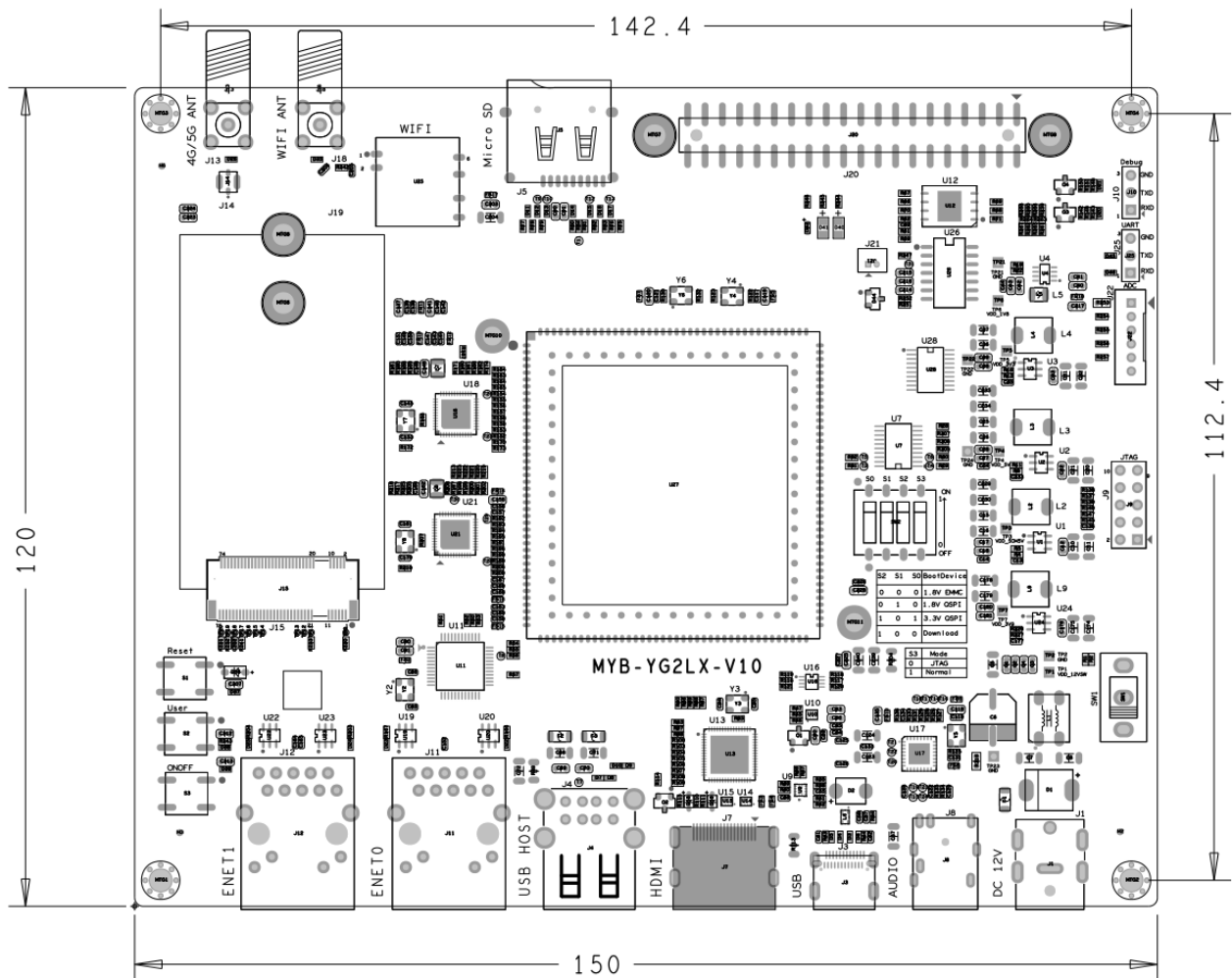
图 4-4 MYB-YG2LX 机械尺寸图 (单位: mm)
