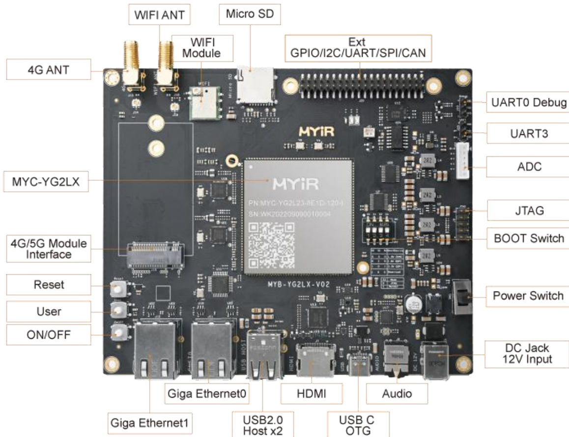
图 4-1 MYD-YG2LX 开发板接口正面图
